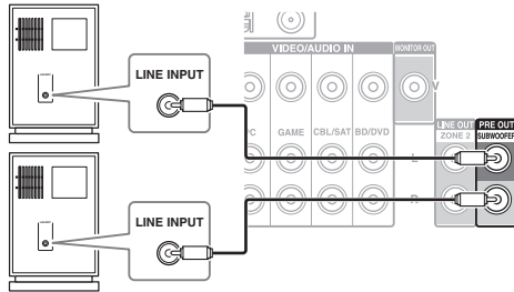
Subwoofer amplifié
